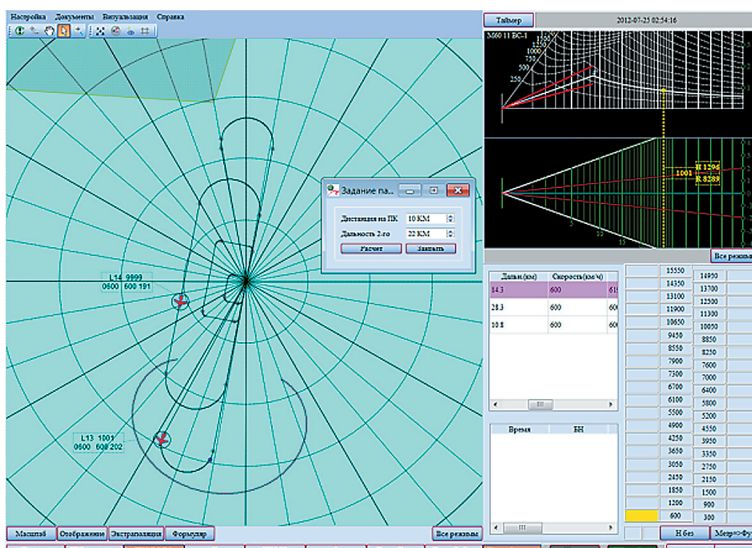
АРМ льотчика-оператора. Задача «Контролю місцезнаходження ЛАК на глісіді»
